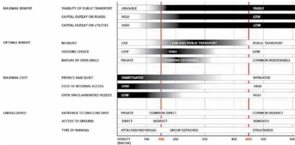
Figure 4.7: Density parameters
